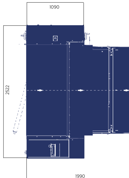
Grundriss KS 601
