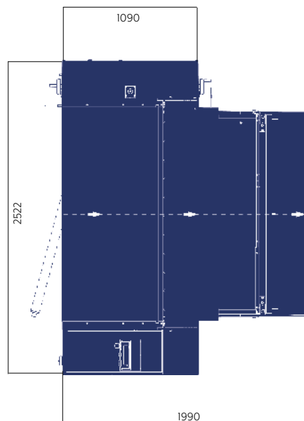
Floorplan KS 601
